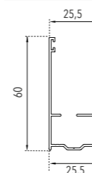
ART. GU60 antvento Guida in alluminio A60 25,5 X 60 mm
